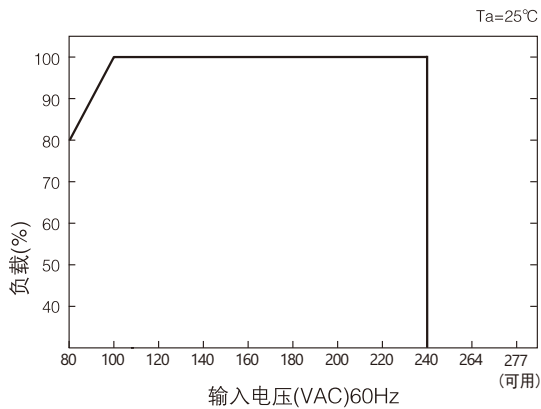
■ 减额输出VS输入电压曲线
