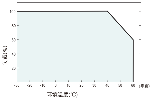
■ 减额曲线
