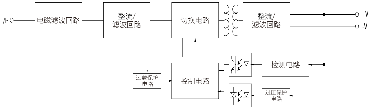
■ 方框图
